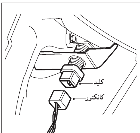
شکل ۱۵۱- تعویض کلید
