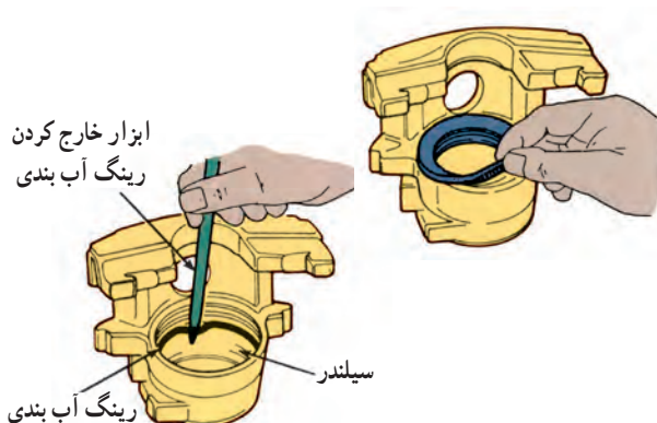
شکل ۱۲۲- قطعات غیر فلزی سیلندر ترمز دیسکی
