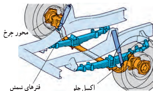
شکل ۳-۱۱ سیستم تعلیق یک پارچه با فنرهای شمش
