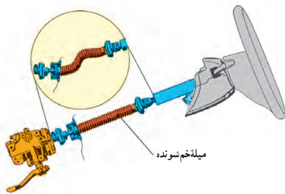
شکل ۱۹-۲ فرمان با میله خم شونده
