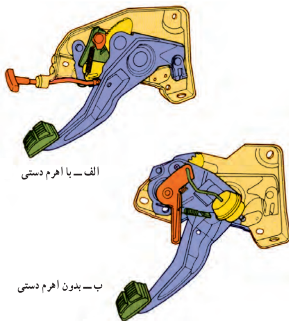
شکل ۴۲-۱ اهرم پای
