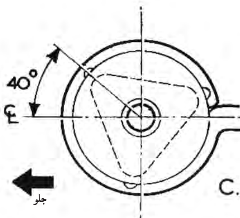
شکل ۳-۷۳ - بوش لاستیکی مثلثی با بوش فلزی مرکزی
