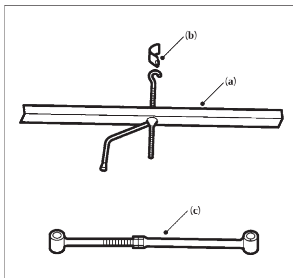
شکل ۳-۱۶۰ - ابزار مخصوص
