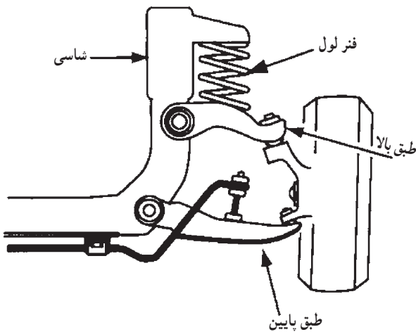
شکل ۳-۵۵ سیستم تعلیق جلو با فنر ماریچ نصب شده روی طبق بالا
