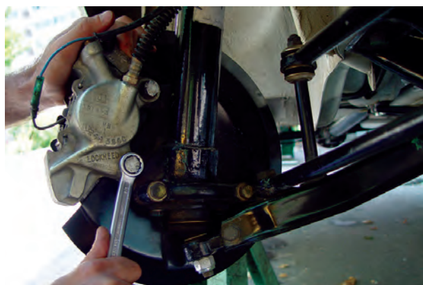
شکل ۳-۷۷ – باز کردن کالیپر ترمز
