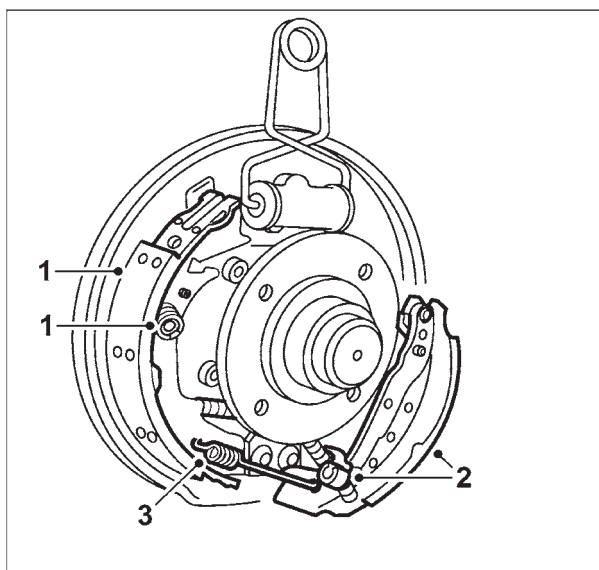
شکل ۹۸-۱- نصب کشک‌ها و متعلقات آنها
