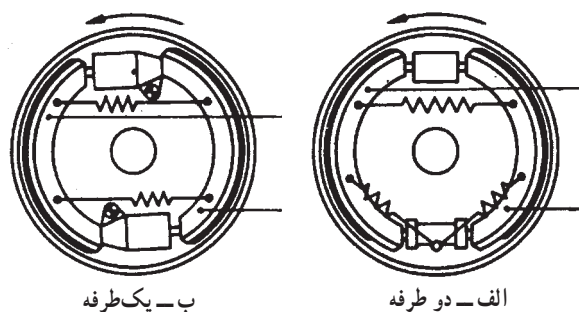
شکل ۱-۳۴ - سیستم ترمز کفشکی با سیلندر
