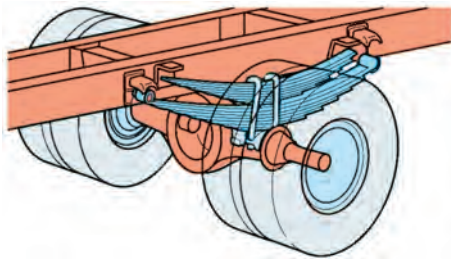
شکل ۱۳-۳ سیستم تعلیق با فنر شمش دبل خودروهای سنگین
