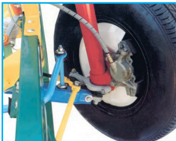
شکل ۱-۳۲ - لوله مایع ترمز انعطاف پذیر
