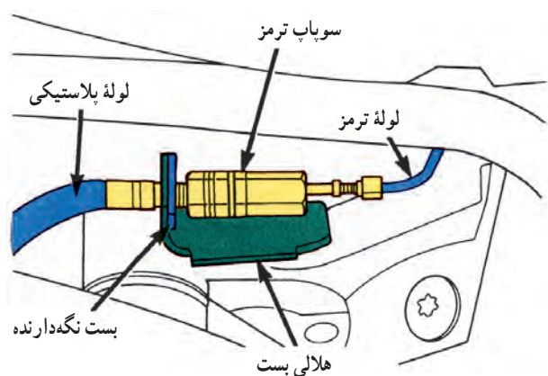
شکل ۸۱-۱- اتصال لوله ترمز
