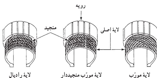
شکل ۳-۲۱۱ - لایه‌گذاری لاستیک‌ها
