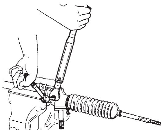
شکل ۸۷-۲- کنترل گشتاور پنیون
