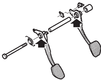
شکل ۱۴۸- اجزای پدال‌ها روی محور پدال
