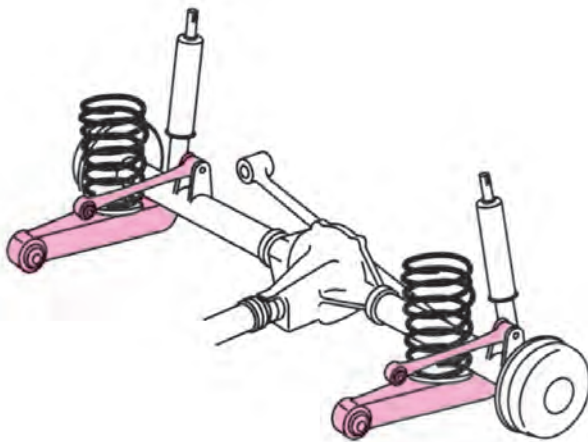
شکل ۴۶-۳ سیستم تعلیق یک پارچه با فنر مارپیچ
