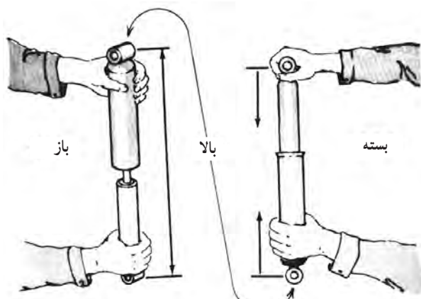
شکل ۳-۴۰ - اصول کار کمک فنر
