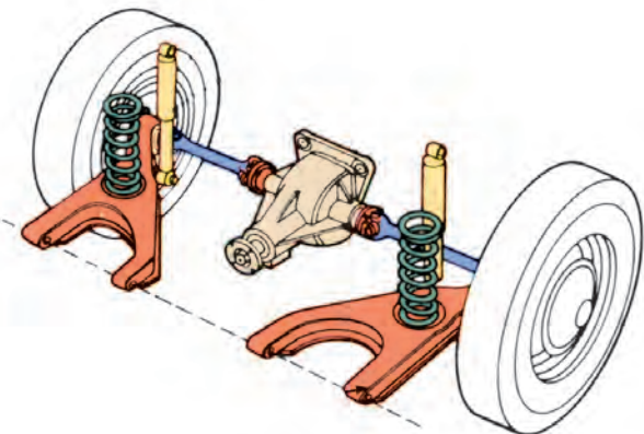
شکل ۴۷-۳ سیستم تعلیق مستقل عقب با چرخ‌های محرک
