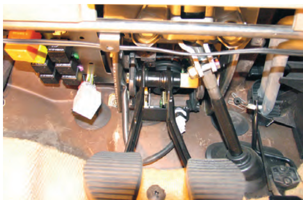
شکل ۱۵۲- کلید چراغ ترمز
