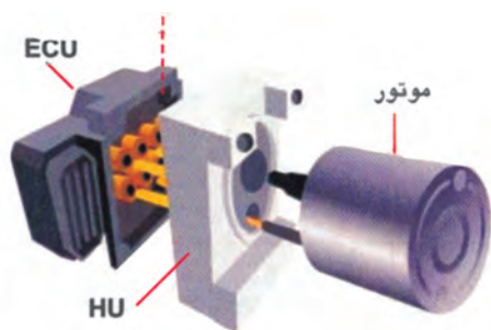
شکل ۱۶۰-۱- موتور
