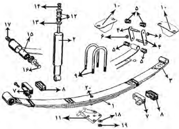
شکل ۴۵-۳ اجزای سیستم تعلیق با فنر شمش چند لایه
