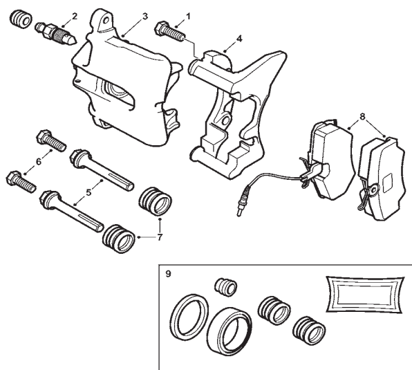
شکل ۱۲۱- اجزای سیستم ترمز
