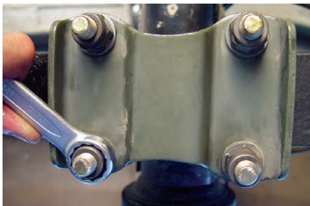
شکل ۳-۶۶- باز کردن مهره‌های کربی‌ها (پیچ‌های U شکل)
