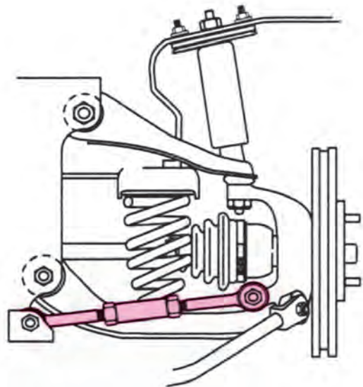
شکل ۳-۵۴ سیستم تعلیق جلو با فنر ماریچ نصب شده
