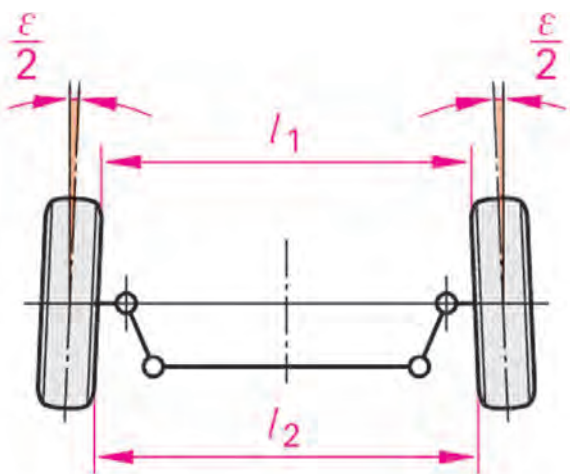
شکل ۲-۲۶ - زاویه تواین (Toe-in)
