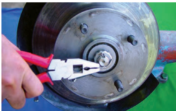
شکل ۳-۹۳ – خارج کردن پین و ضامن مهره تویی
