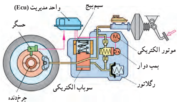
شکل ۱۶۳-۱- سیستم ترمز ضد قفل (ABS)
