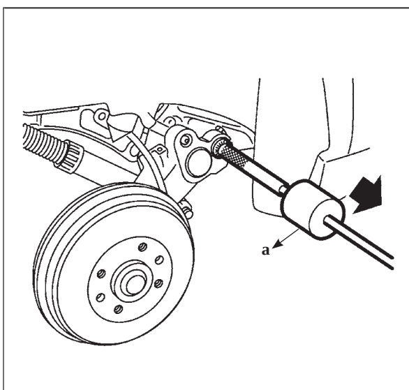
شکل ۳-۱۶۵ بیرون کشیدن میل موج‌گیر
