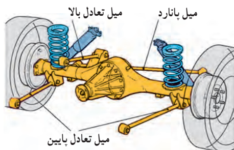
شکل ۳-۱۲ سیستم تعلیق یک پارچه با چرخ های محرک
