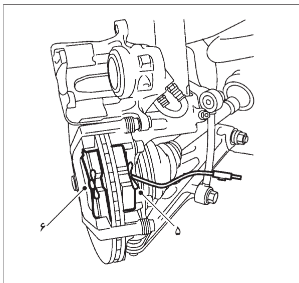
شکل ۱۱۵- نصب لنت‌ها
