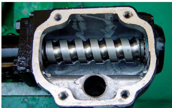
شکل ۶۴-۲- ماریچ فرمان
