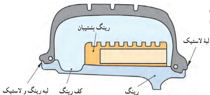
شکل ۳-۲۱۰ - لاستیک تخت با رینگ پشتیبان
