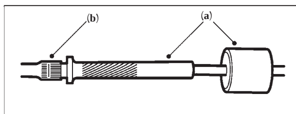
شکل ۳-۱۶۶ نصب ابزار و چکش لغزان بر روی میل موج‌گیر
