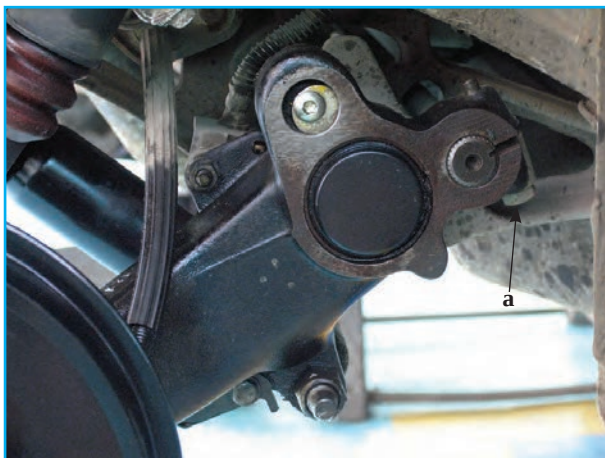
شکل ۳-۱۶۴ باز کردن بست‌های میله موج‌گیر
